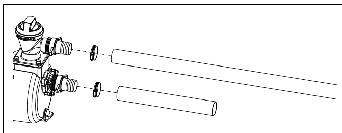
Figura 4-7. Conexión de las mangueras
