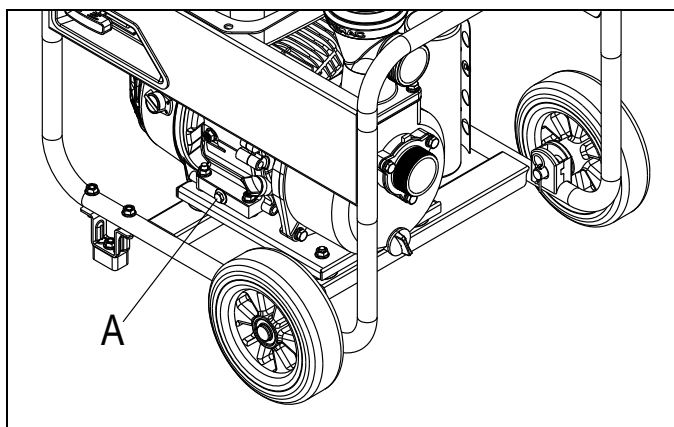
Figure 6-4. Bouchon de vidange d'huile du modèle ST20
