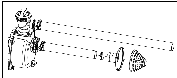
Figura 4-8. Conexión del filtro
