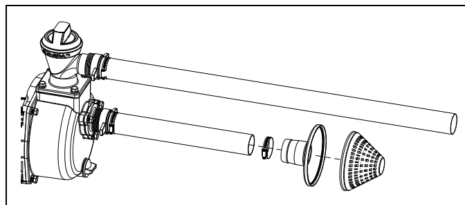
Figure 4-8. Fixation du filtre
