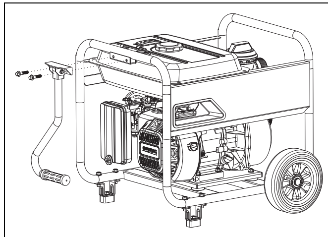
Figure 4-2. Fixation de la poignée
