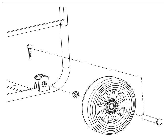
Figure 4-3. Fixation des roues
