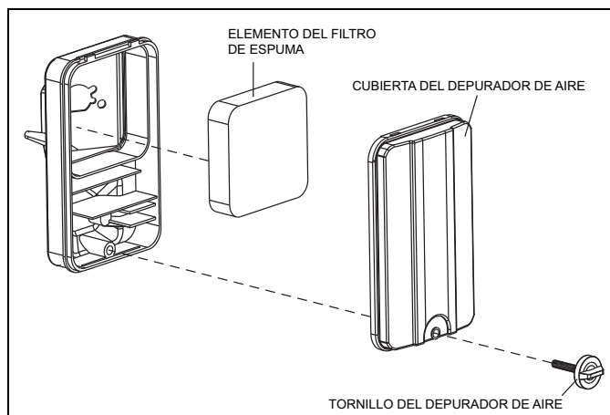
Figura 6-6. Servicio del depurador de aire ST20
