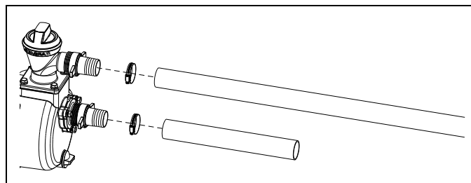
Figure 4-7. Fixation des tuyaux
